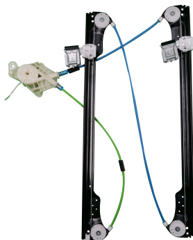
POWER WINDOW LEFT ALZACRISTALLI ELETTRICO SX
