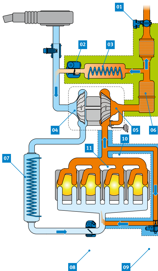
Układ recykulacji spalin (schemat)
