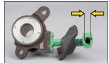
Figur 4: LuK CSC 510 0137 10 hydraulisk tilkobling 12.2 mm
