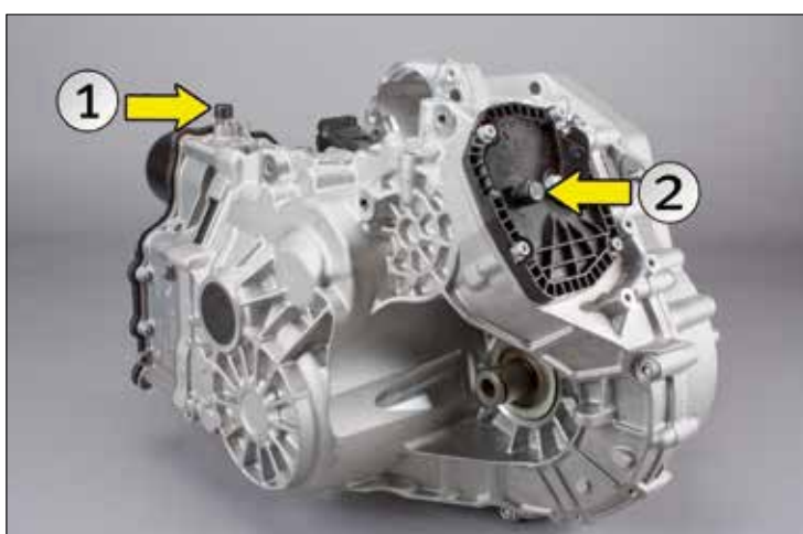
Figur 1: Direktekoblingsgirakasse med ventilerende hetter for mekatronikk (1) og girakasse (2)
