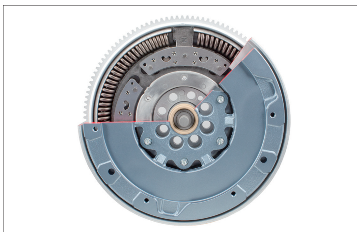
Foto1: Dwumasowe koło zamachowe z odśrodkowym tłumikiem drgań typu wahadłowego
