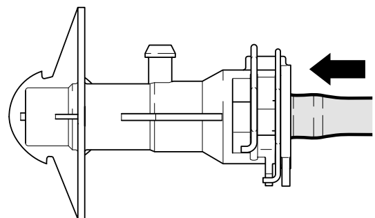
Foto 4: Złącze wsunięte, klipsy zapięte, odpowietrznik zamknięty
