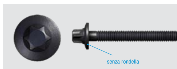
Fig. 2_Nuova vite senza rondella (OE-Nr. 65 07 937)
