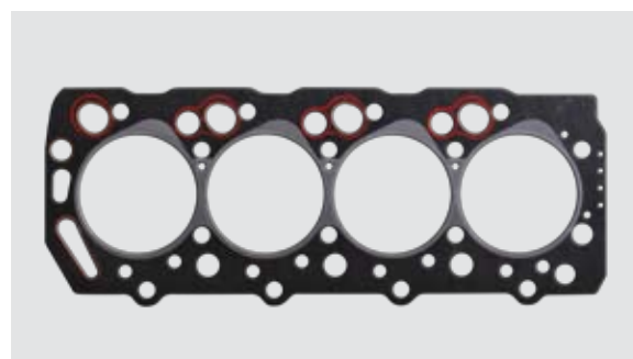
Rys. 2_61-52252-30 (nowa wymienna uszczelka głowicy cylindra)
