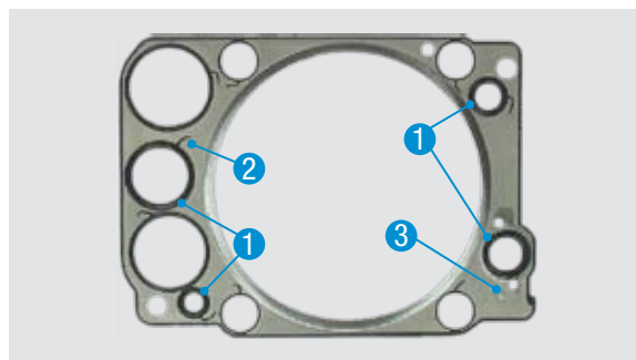
Уплотнительная поверхность с выфрезерованными пазами 61-37190-10
