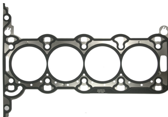
Ilustración_Empaquetadura de culata con N° Reinz 61-36225
