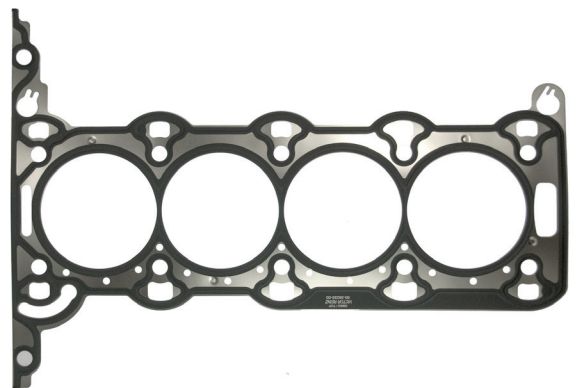
Figura_Guarnizione della testata con Reinz n. 61-36225
