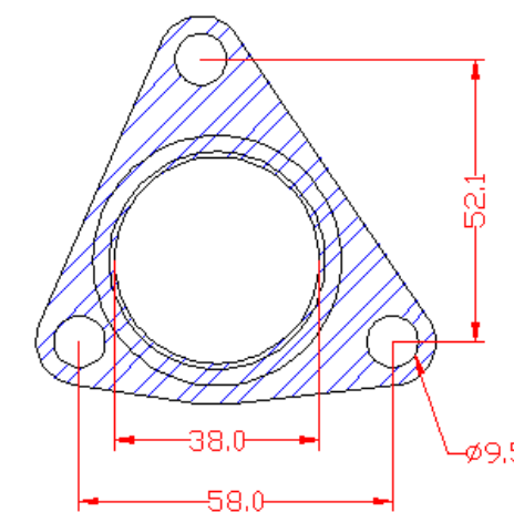
Cotes du joint
