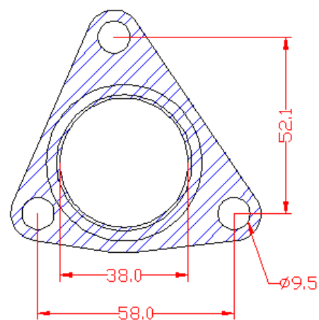
Cotas de la junta
