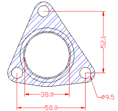
Maßangaben der Dichtung
