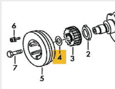
sl. 2 Položaj za montažu
