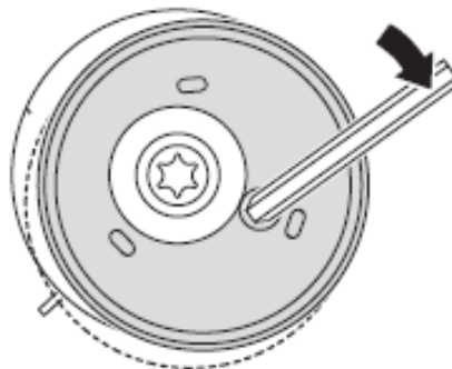
Bild 2 Spännrulle utan låsstift
