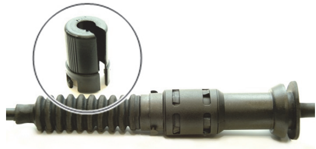
Abb. 4: Sicherung entfernt
