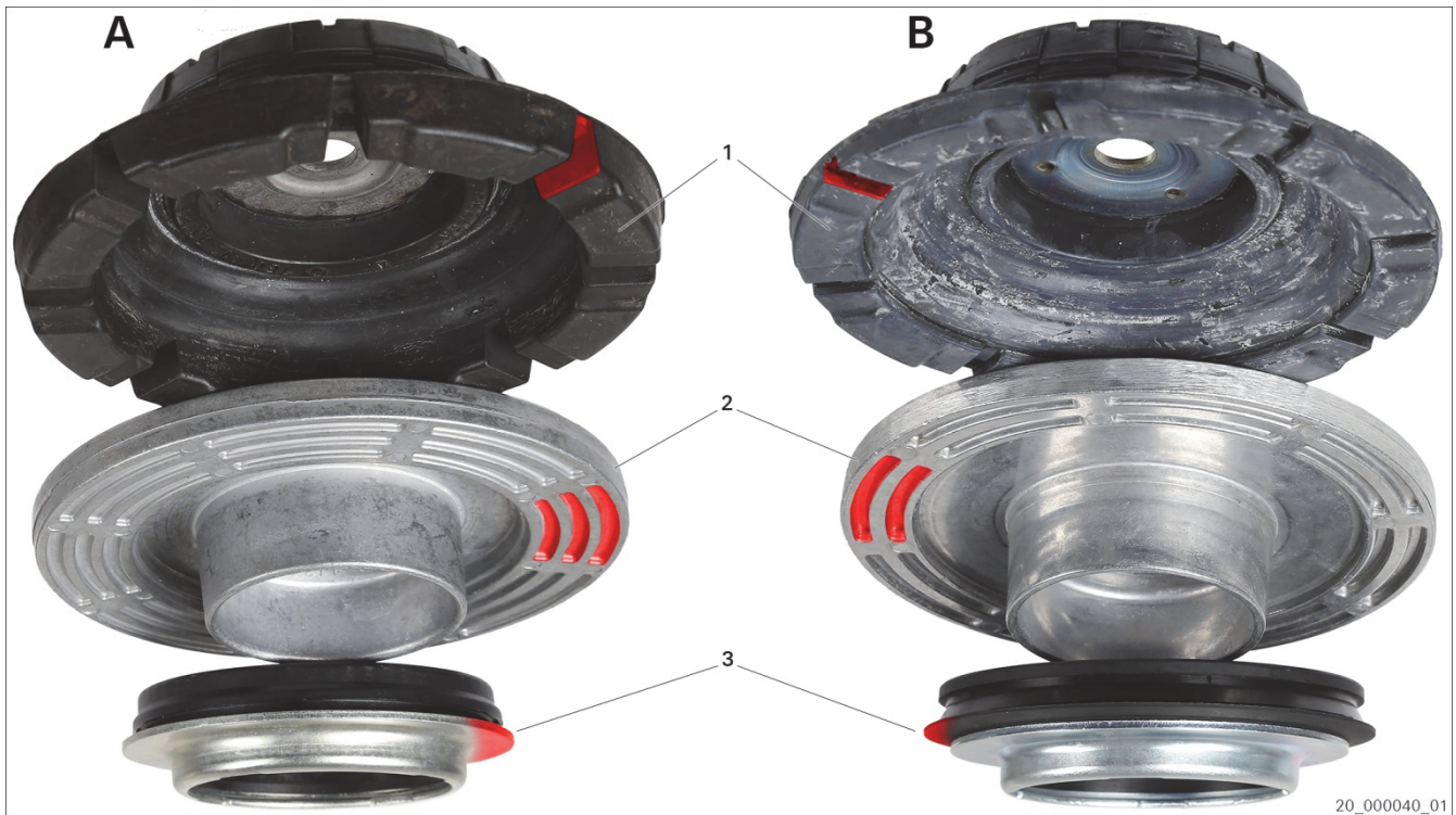
Fig. 1: Fjærbeinstøttelager variant A/B
