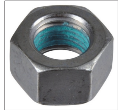
Abb. 2: Mutter M14x1,5 mit chemischer Gewindesicherung
