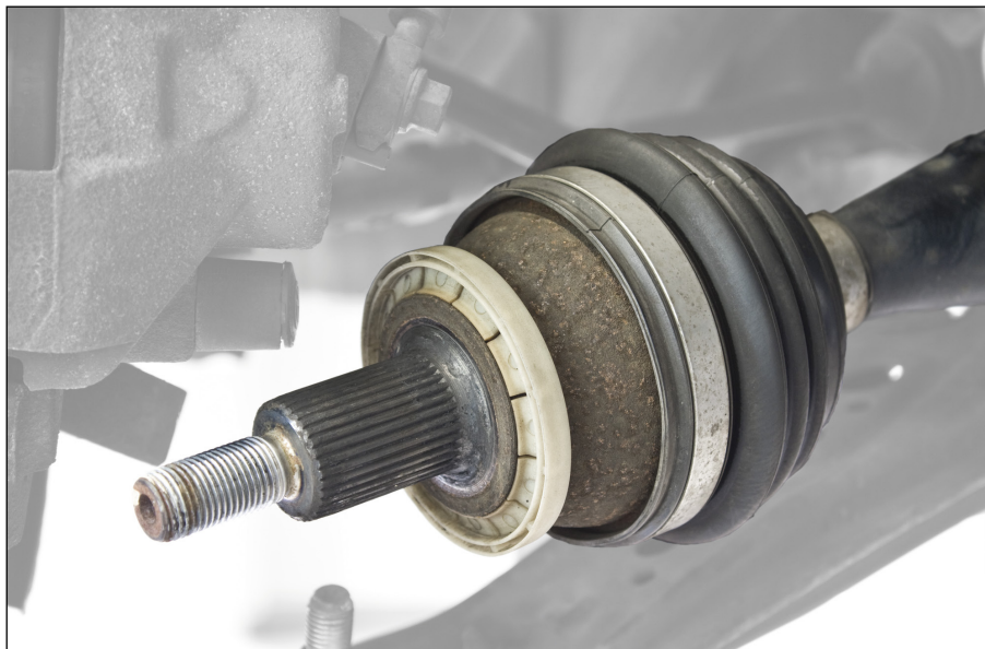
Figur 1: Tetningsringene kan skille seg fra hverandre når det gjelder utseende og farge!
