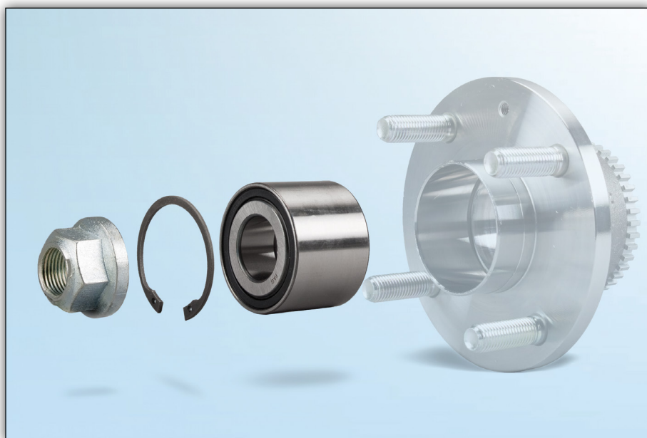
Figur 1: FAG-hjulkulelagersettet 713 6448 00 som en reparasjonsløsning – det er ikke nødvendig å skifte ut hjulnavet.
