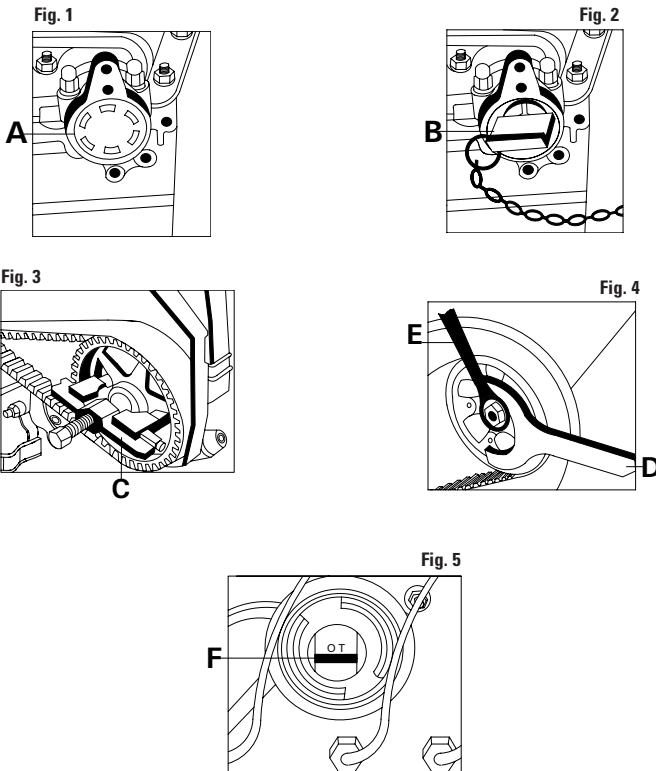
FIGURA 1 Extraer el tapón del cabezal de motor derecho A. FIGURA 2 Insertar la herramienta especial de inmovilización de árbol de levas B. FIGURA 3 Extractor de poleas de árbol de levas C. FIGURA 4 Insertar la herramienta especial D para mantener a la correa en tensión entre los engranajes y luego afloje los tornillos de poleas de ambos arboles de levas utilizando la herramienta E. FIGURA 5 Verificar la correcta alineación de la marca de puesta a punto F quitando la tapa de llenado del aceite. FIGURE 1 Enlever le bouchon de la culasse droite A. FIGURE 2 Introduire les outils appropriés de blocage arbres à cames B. FIGURE 3 Extracteur poulies d'arbre à cames C. FIGURE 4 Introduire l'outil approprié D pour maintenir l'engrenage sous tension et desserrer les vis des poulies arbre à cames en utilisant l'outil E. FIGURE 5 Contrôler le correct alignement du point de repère de phase F en enlevant le bouchon de remplissage d'huile.
