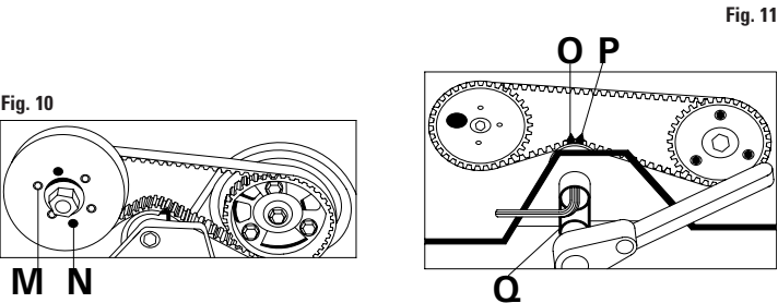
FIGURA 10 Extraer el amortiguador de vibraciones de la polea de la bomba de inyección por medio de los tornillos M. Jamás afloje el tornillo N. FIGURA 11 Aflojar el tornillo de fijación del tensor de correa. Girar el tensor de la correa en sentido contrario a las agujas del reloj hasta que los indicadores O y P estén alineados. Por último, apriete el tornillo de fijación del tensor utilizando la herramienta específica Q.
