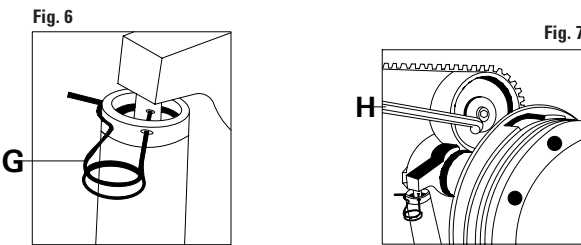
FIGURA 6 Insertar la herramienta para inmovilización del tensor de correa G. FIGURA 7 Girar el tensor de correa en sentido contrario a las agujas del reloj, utilizando para ello la llave hexagonal H, hasta alcanzar la tensión correcta. Por último, desmonte la herramienta de inmovilización G.
