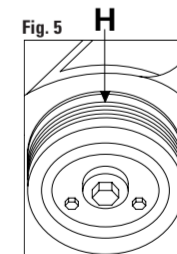
FIGURA 4 Marcas de referencia sobre el volante de inercia del motor. Verificar la correcta alineación de las marcas de fase G. FIGURA 3 Marcas de referencia sobre el volante de inercia del motor. Verificar la correcta alineación de las marcas de fase F. FIGURA 5 Verificar la correcta alineación de la marca de puesta a punto H.
