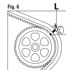
FIGURA 6 Controllare il corretto allineamento delle tacche di fase I con il bullone L.
