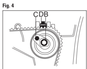
FIGURA 2 Allentare il bullone di bloccaggio B e ruotare in senso orario il tendicinghia sull'eccentrico di registro C, ed allineare l'indicatore D nella zona di controllo; Serrare, quindi, il dado di bloccaggio B. Tensione alla temperatura di -20° C. FIGURA 3 Allentare il bullone di bloccaggio B; ruotare in senso orario il tendicinghia sull'eccentrico di registro C, ed allineare l'indicatore D nella zona di controllo; serrare quindi il dado di bloccaggio B. Tensione alla temperatura di 20° C. FIGURA 4 Allentare il bullone di bloccaggio B; ruotare in senso orario il tendicinghia sull'eccentrico di registro C, ed allineare l'indicatore D nella zona di controllo; serrare, quindi, il dado di bloccaggio B. Tensione alla temperatura di 50° C.
