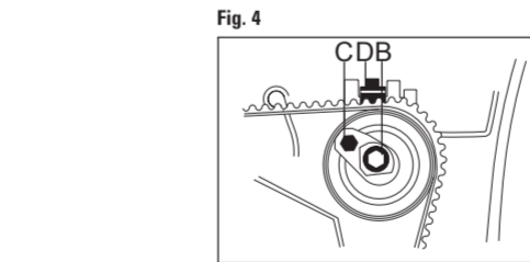
FIGURA 2 Aflojar el tornillo de fijación B, girar el tensor de correa sobre el excéntrico de regulación C en sentido de las agujas del reloj, alineando el indicador D en la zona de control. Luego vuelva apretar la tuerca de fijación B. Tensión a la temperatura de -20° C.
