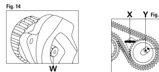
FIGURA 14 Allentare il bullone di bloccaggio W posto sul retro del tendicinghia del contralbero. FIGURA 15 Allentare il bullone di bloccaggio X del tendicinghia del contralbero ed inserire l'apposito attrezzo di tensionamento Y; allineare l'indicatore mobile Y con la tacca di fase Z; serrare, quindi, il bullone di bloccaggio W.
