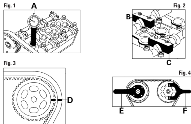
FIGURA 1 Inserire l'apposito attrezzo di comparazione A, sul cilindro N° 1. FIGURA 2 Smontare il cappelotto: del 2° cilindro lato scarico dell'albero a camme (per modello JTS); del 2° cilindro lato aspirazione dell'albero a camme (per modello Delta); del 3° cilindro lato aspirazione dell'albero a camme (per tutti i modelli); del 3° cilindro lato scarico dell'albero a camme (per modello Delta); del 4° cilindro lato scarico dell'albero a camme (per modello Barchetta); ed inserire gli appositi attrezzi bloccaggio B e C. FIGURA 3 Controllare il corretto allineamento delle tacche di fase D. FIGURA 4 Attrezzi per il mantenimento della tensione dell'albero a camme E ed F.
