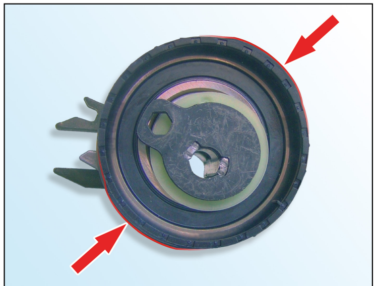
Figur 1: 531 0564 30 (visning forfra)
