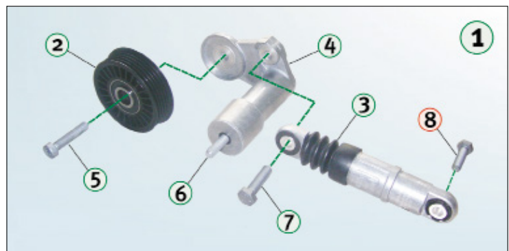
Figur 1: Detaljert illustrasjon av 534 0014 10 inkludert alle komponenter
