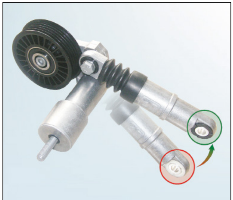
Figur 2: 534 0014 10 - Versjon viser både sort og hvit plastføring på hydraulisk demper
