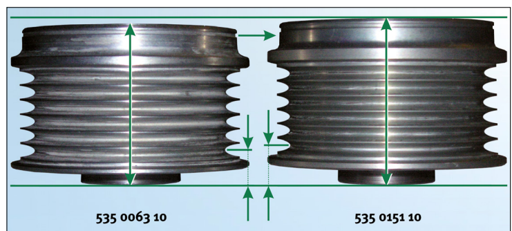
Figur 3: Skille mellom INA-friløpsremskive OAP 535 0063 10 (VALEO) og 535 0151 10 (DENSO)
