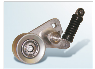
Figur 2: 534 0340 10 - nåværende utforming
