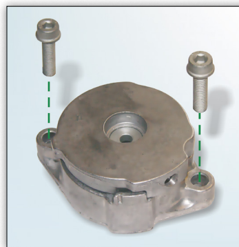
Figur 1: INA utforming med to M8x35 bolter
