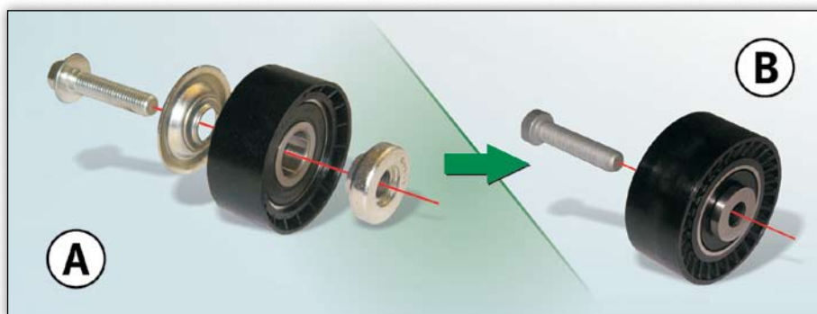
Rolka prowadząca 532 0433 10, wersja stara (A) i nowa (B)
