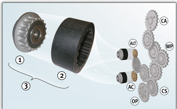
Figur 1: Friløpremskive med fleksibel koplingsmuffe og tanndrev
