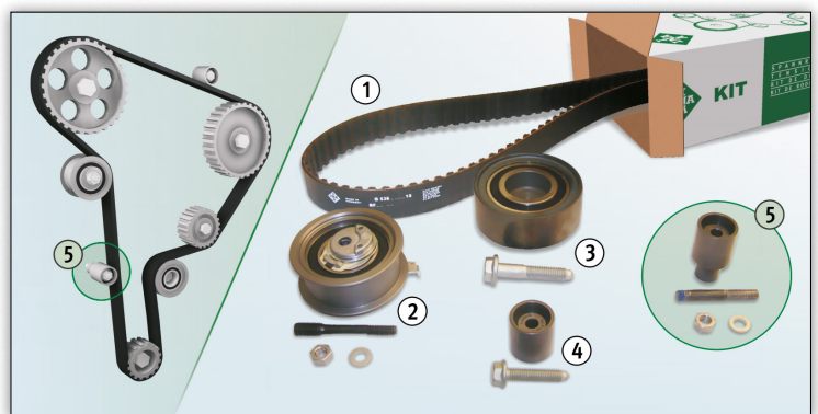
Figur 1: Drev-diagram 1.9 TDI/SDI og pakkeinnhold for SETT 530 0361 10/530 0082 10
