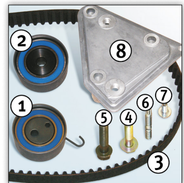
Figur 2: Pakkeinnhold: 530 0492 10
