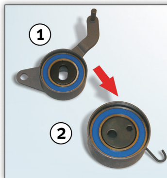
Figur 1: Erstattet spennrulle 531 0166 20 (1) og dens etterfølger 531 0819 10 (2)
