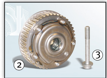
Figur 2: Kamakselering for uttakssiden 427 1005 10 og sentral bolt 41301*
