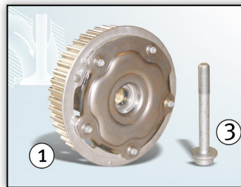
Figur 1: Kamakselering for inntakssiden 427 1004 10 og sentral bolt 41301*
