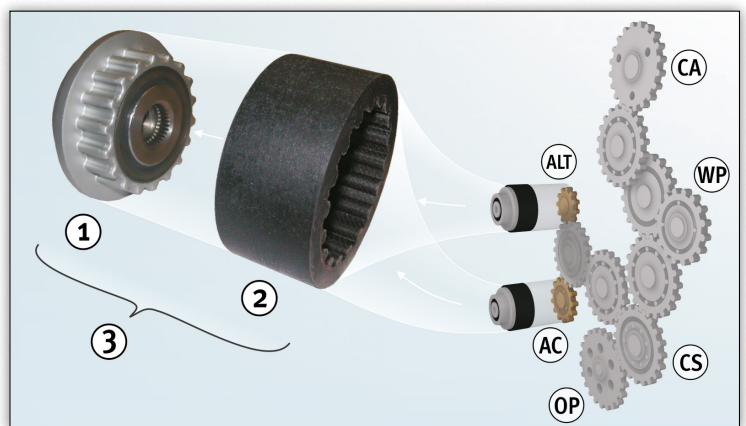
Figur 1: Friløpremskive med fleksibel koplingsmuffe og tanndrev
