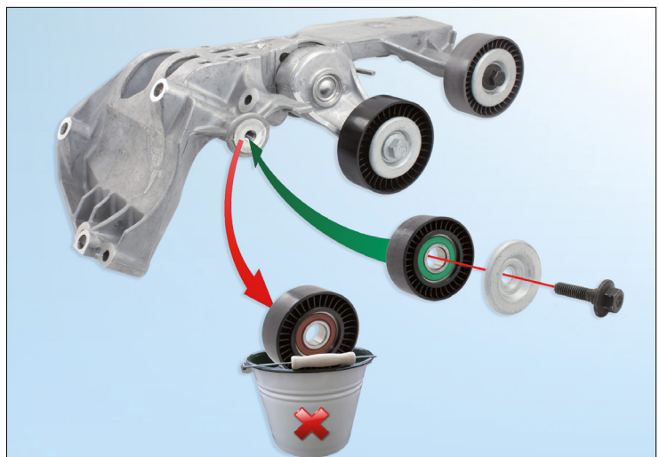
Figur 1: Spennenhetsmontering 534 0243 10
