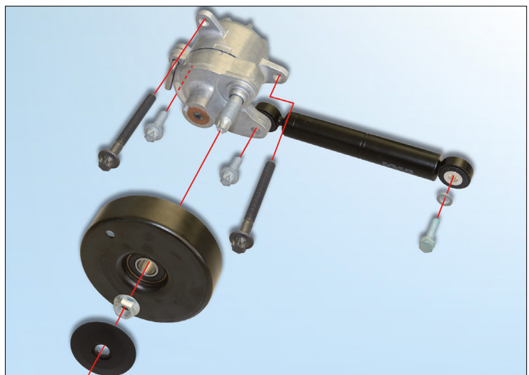
Figur 1: 533 0116 10 – INA reparasjonssett til monterte drev inkludert festeskruer
