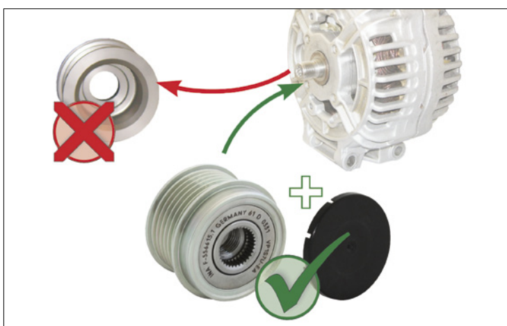
Foto1: Wymiana sztywnego koła pasowego na wolne koło alternatora
