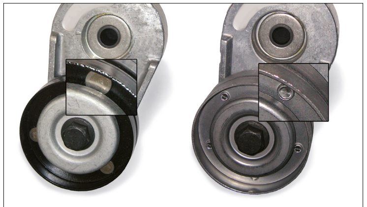
Figur 1: Detaljert visning over rullene i den tidligere utformingen (venstre) og den nye utformingen (høyre)
