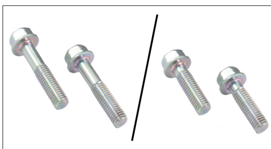
Figur 4: Venstre, tidligere M8x40 mm skruer. Høyre, nye M8x30 mm skruer.
