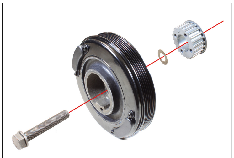
Figur 1: veivaksels vibrasjonsdemper med sentral skruer til veivaksel og diamantskive
