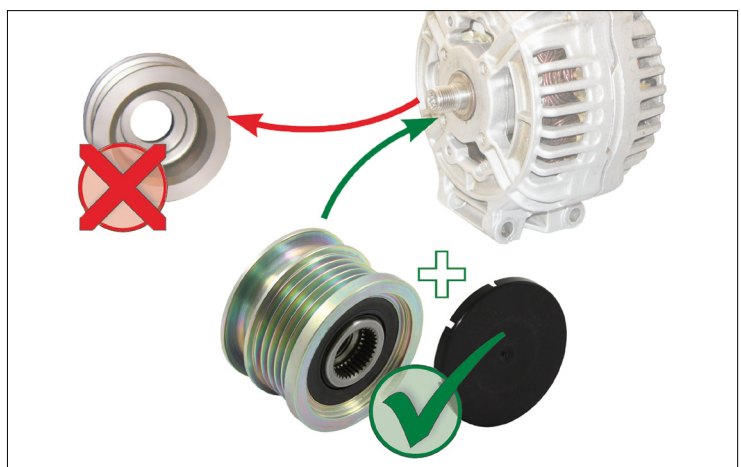
Figur 1: Skifte fra en stiv remskive til en friløpsremskive OAP
