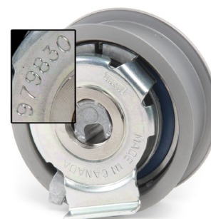
Foto 2: 531 0851 10 – Nowa rolka napinająca (979830)
