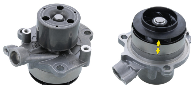
Foto 1: Pompa wody 538 0983 10 z przestawianą aperturą wirnika
