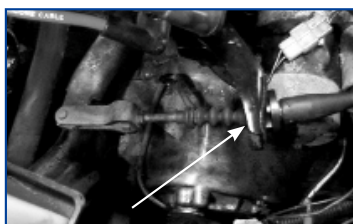
Clutch cable seizure
