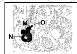
Figura 11: Montare la dima albero motore inserendo il perno M dell'attrezzo N nel foro O.
