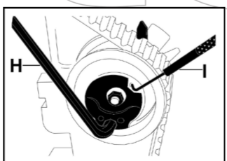
Figura 7: Allentare il dado del tenditore, ruotare il tenditore in senso antiorario con l'attrezzo H e inserire l'attrezzo di blocco I.
