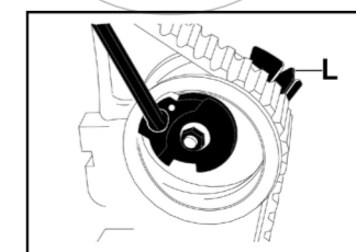
Figura 10: Ruotare il tenditore in senso orario e portare l'indicatore mobile L nella posizione di tensione, serrare quindi il dado di fissaggio.
