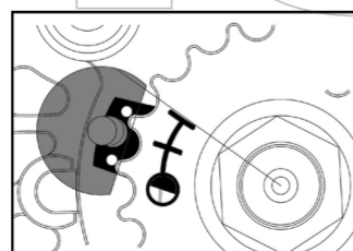
Figura 6: Ruotare in senso orario di due giri l'albero motore e reinserire i vari attrezzi per la verifica della corretta fasatura. Verificare che la puleggia della pompa alta pressione sia posizionata come illustrato.
