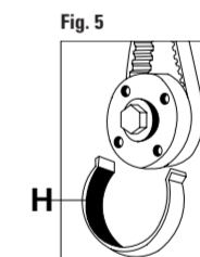
FIGURA 4 Inserire l'apposito attrezzo di bloccaggio del volano G. FIGURA 5 Inserire l'apposito attrezzo di bloccaggio della cinghia di distribuzione H. FIGURA 6 Controllare il corretto allineamento delle tacche di fase I.
