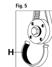
FIGURA 4 Insertar la herramienta de inmovilización del volante motor G. FIGURA 5 Insertar la herramienta específica para inmovilizar la correa de distribución H. FIGURA 6 Verificar la correcta alineación de las marcas de puesta en fase I.
