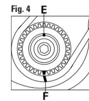
FIGURA 4 Verificar la correcta alineación de las marcas de puesta en fase E y F.
