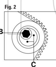
FIGURA 2 Allentare il bullone di bloccaggio B e ruotare in senso antiorario il tendicinghia sull'eccentrico di registro C fino alla corretta tensione; serrare quindi il bullone di bloccaggio B.
