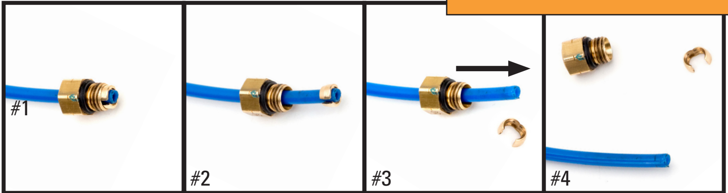
#2 向上沿管路移动螺纹部分，移开并取下卡头
