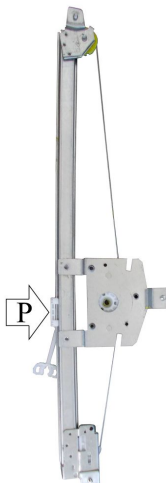
POWER WINDOW LEFT ALZACRISTALLI ELETTRICO SX
